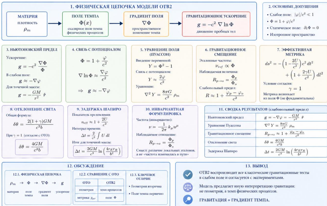
Рис.1. ОТВ2 слабопольный предел и гравитационные тесты.
