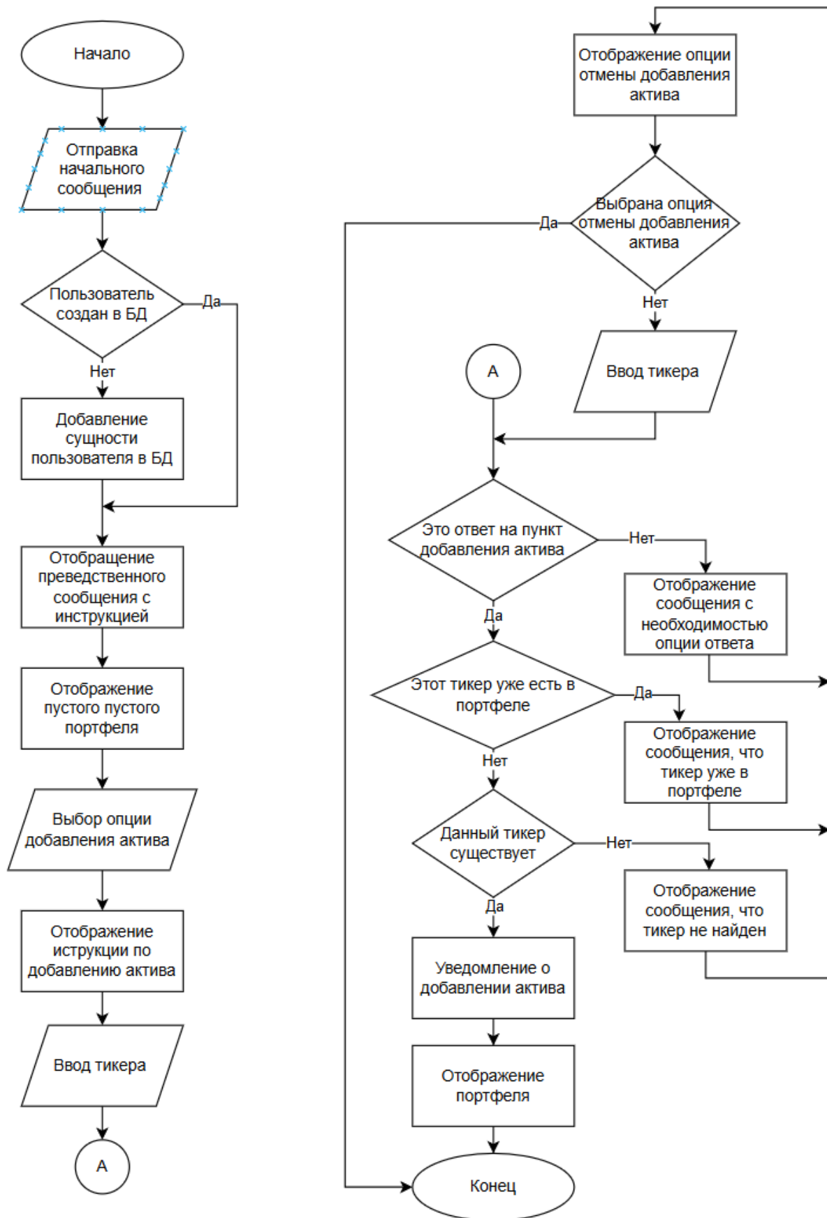
Рис. 2. Блок-схема алгоритма добавления актива
