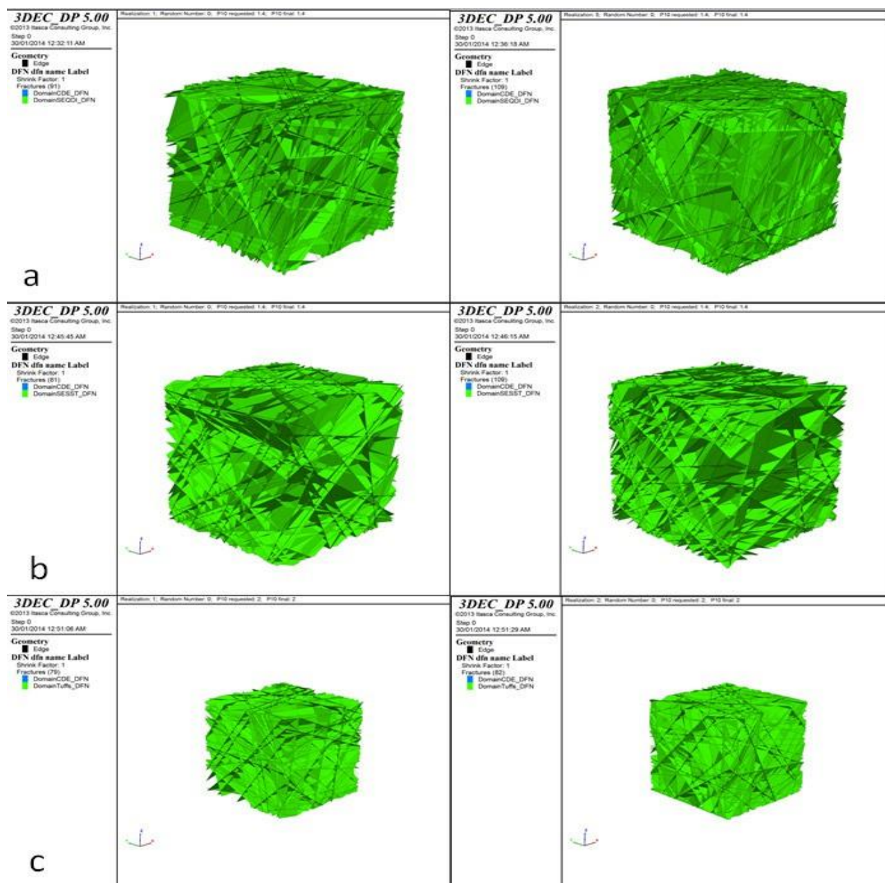
Рисунок 1.2 Примеры СДТ: (а) кварцевых диоритов, (б) отложений и (с) туфов.
