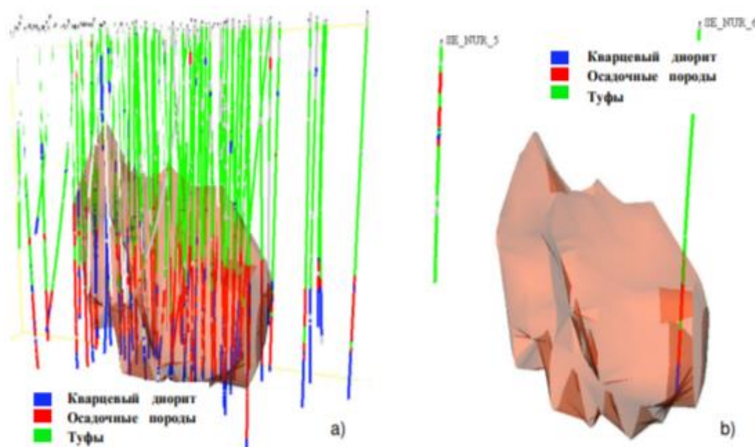
Рисунок 1.1 Примеры ДСТ построенные для интрузивной брекчии (a) и кварцевого диорита (b)
