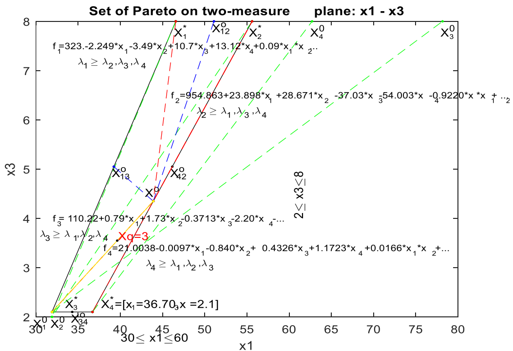
Рис. 1. Допустимое множество точек S в координатах x_1, x_3 . Множество точек, оптимальных по Парето, S^0 \subset S , ограничено точками X_1^*, X_2^*, X_3^*, X_4^* , и локальное S_1^0 между X_1^*, X_{13}^0, X^0, X_{12}^*, X_1^* в двухмерной системе координат \{x_1, x_3\} .
