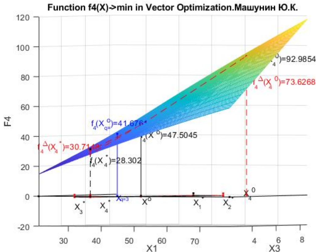
Рис. 9.k3. Функция f_4(X) с приоритетом третьего критерия в двухмерной системе координат x_1, x_3 и геометрическая интерпретация функции f_4(X) в системе координат x_1, x_2, x_3, x_4
