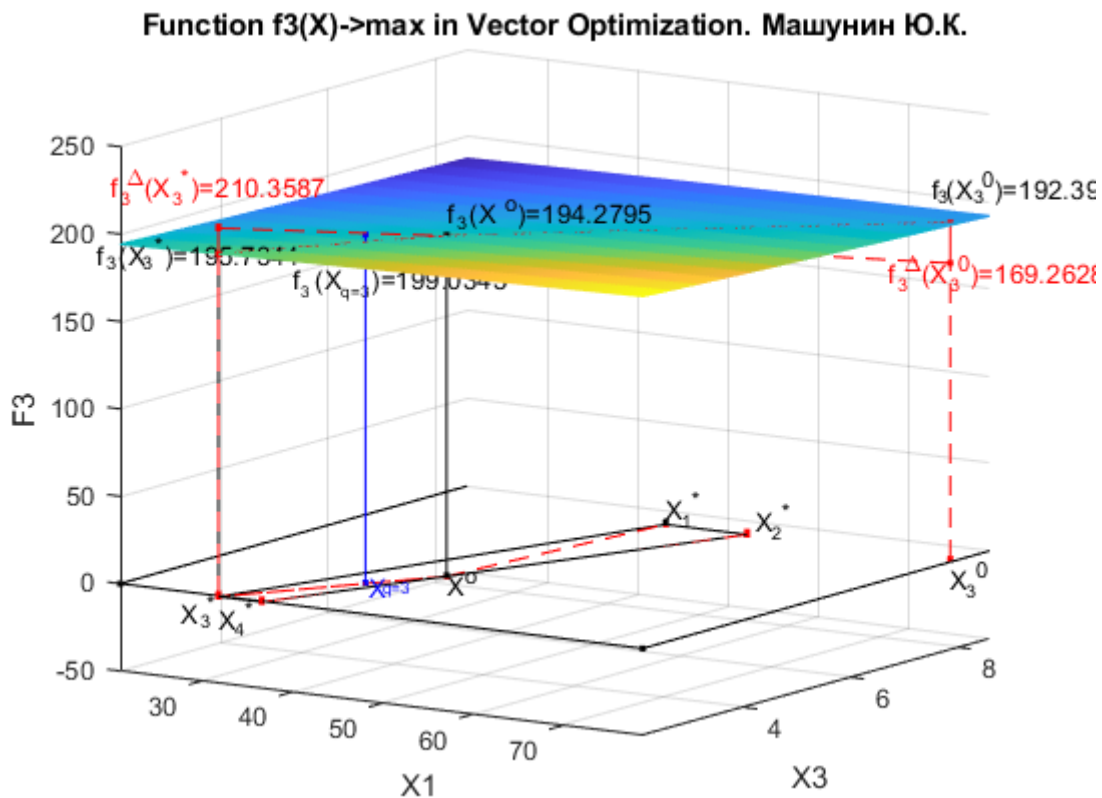
Рис. 8.k3. Функция f_3(X) с приоритетом третьего критерия в двухмерной системе координат x_1 x_3 и геометрическая интерпретация функции f_3(X) в системе координат x_1 x_2 x_3 x_4
