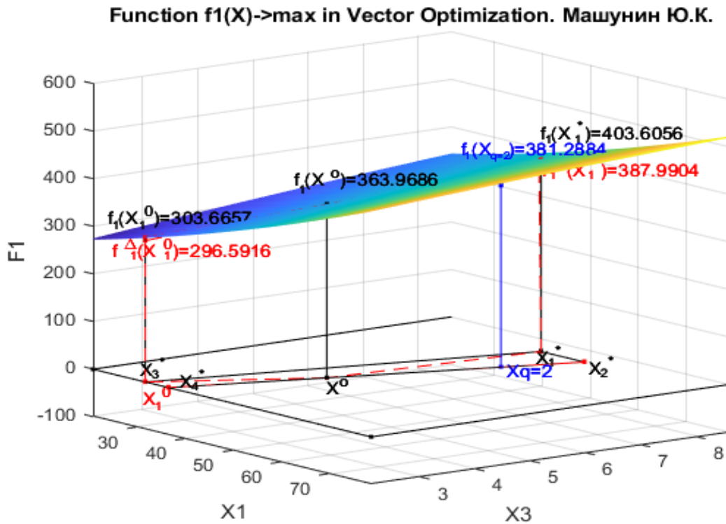
Рис. 6k2. Функция f_1(X) с приоритетом второго критерия в двухмерной системе координат x_1 x_3 и геометрическая интерпретация функции f_1(X) в системе координат x_1 x_2 x_3 x_4
