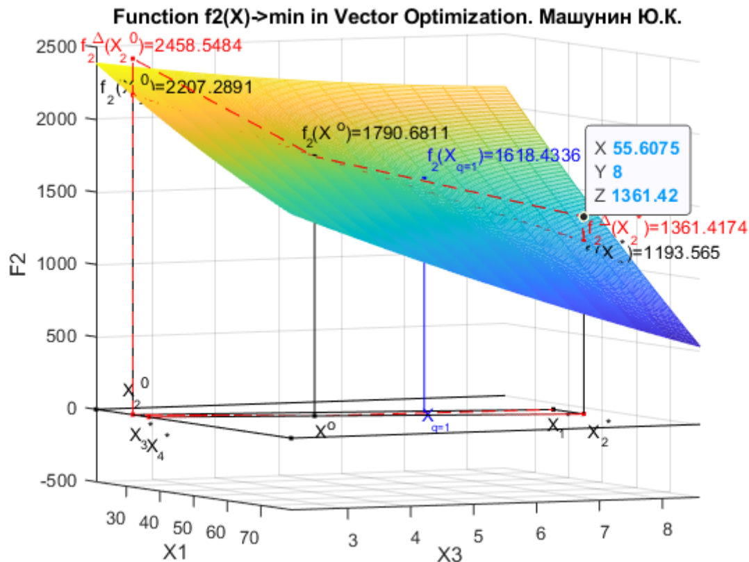
Рис. 7.k1. Функция f_2(X) с приоритетом первого критерия в двухмерной системе координат x_1, x_3 , геометрическая интерпретация функции f_2(X) - координаты x_1, x_2, x_3, x_4
