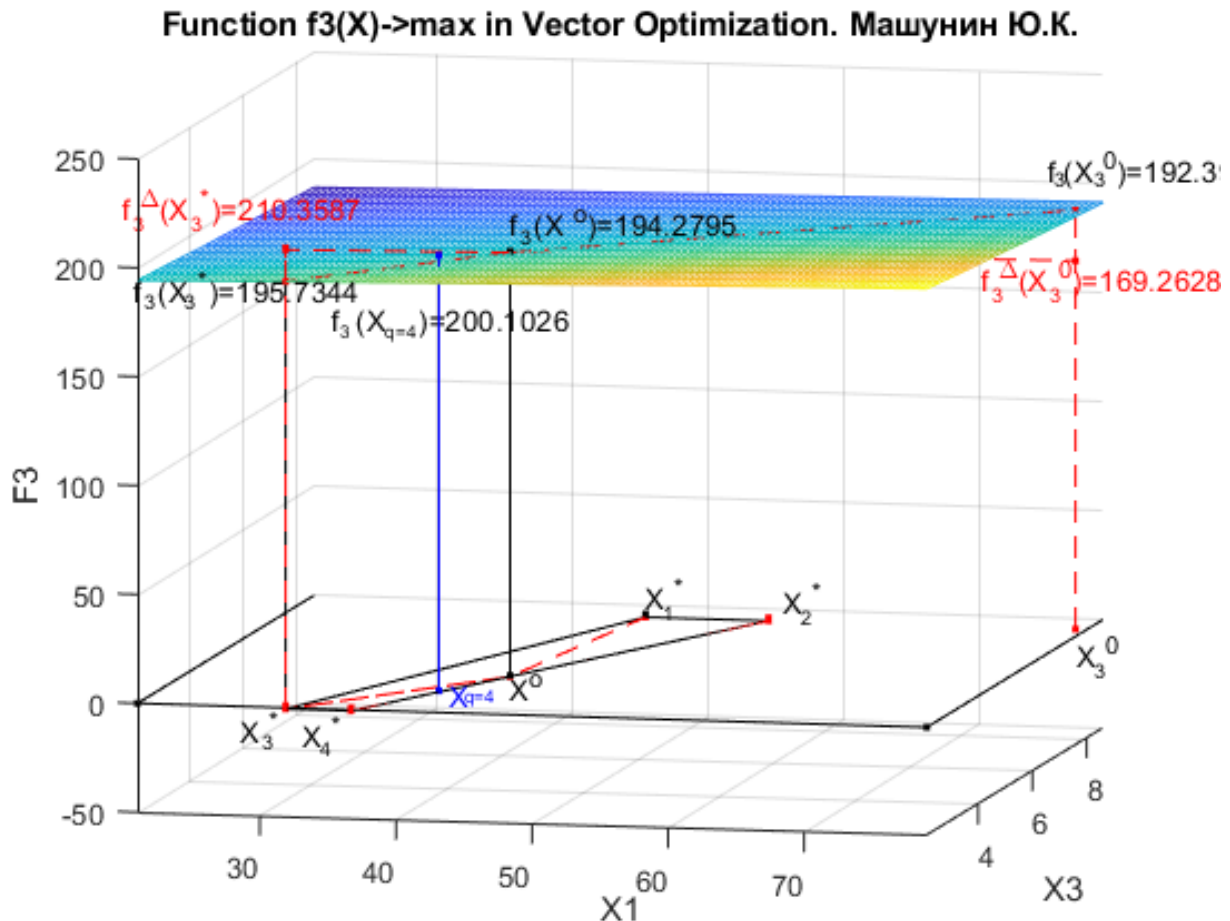
Рис. 8.k4. Функция f_3(X) с приоритетом четвертого критерия в двухмерной системе координат x_1, x_3 и геометрическая интерпретация функции f_3(X) в системе координат x_1, x_2, x_3, x_4
