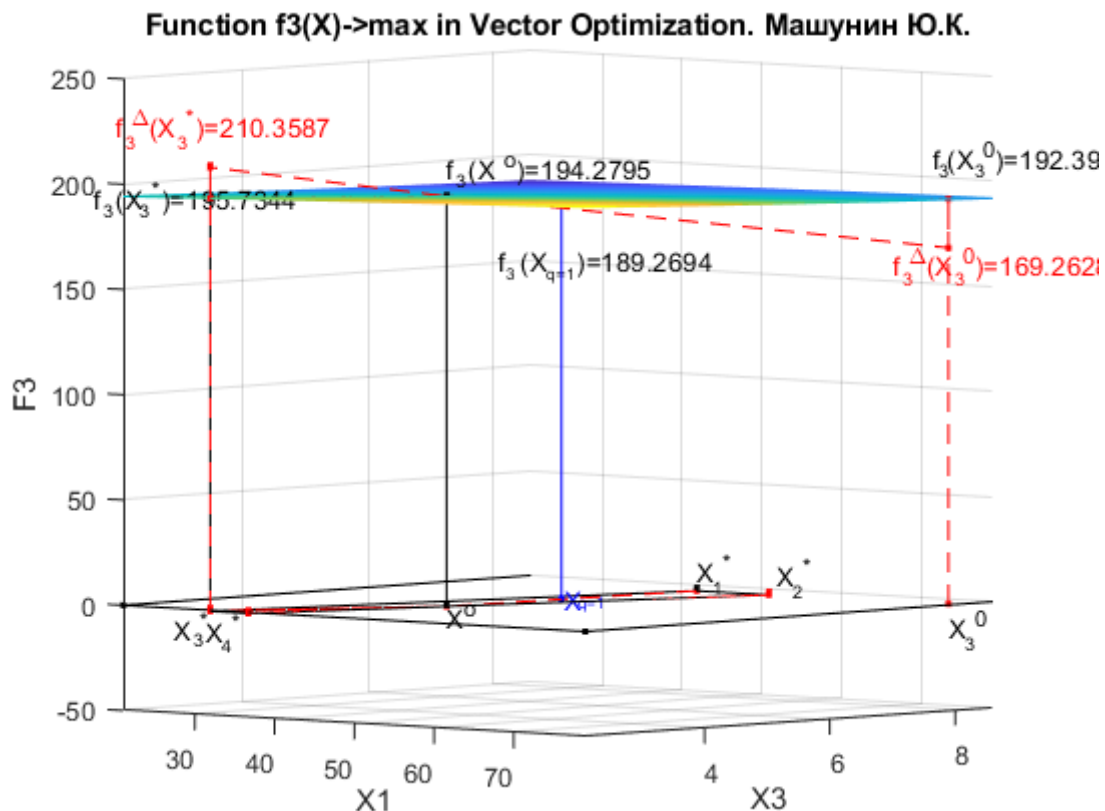
Рис. 8.k1. Функция f_3(X) с приоритетом первого критерия в двухмерной системе координат x_1, x_3 , геометрическая интерпретация функции f_3(X) в системе координат x_1, \dots, x_4 .
