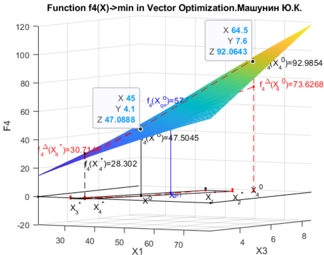
Рис. 9.k1. Функция f_4(X) в двухмерной системе координат x_1, x_3 и геометрическая интерпретация функции f_4(X) с приоритетом первого критерия в системе координат x_1, x_2, x_3, x_4
