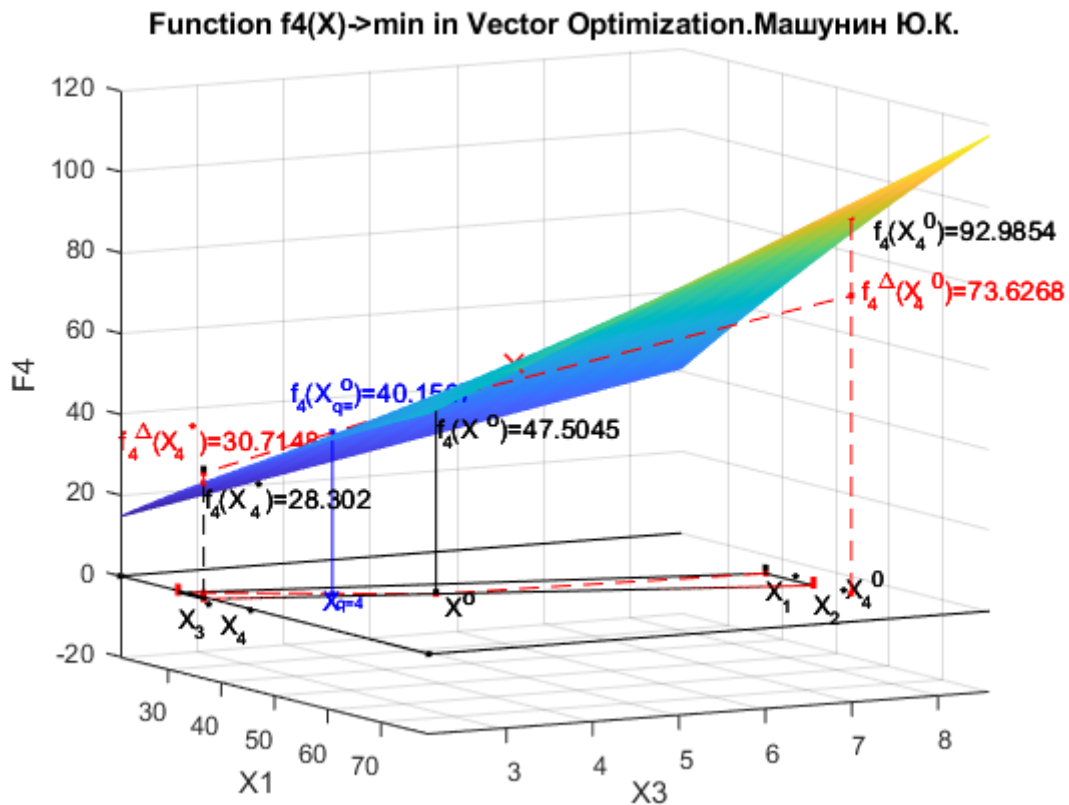
Рис. 9.k4. Функция f_4(X) с приоритетом четвертого критерия в двухмерной системе координат x_1 x_3 и геометрическая интерпретация функции f_4(X) в системе координат x_1 x_2 x_3 x_4
