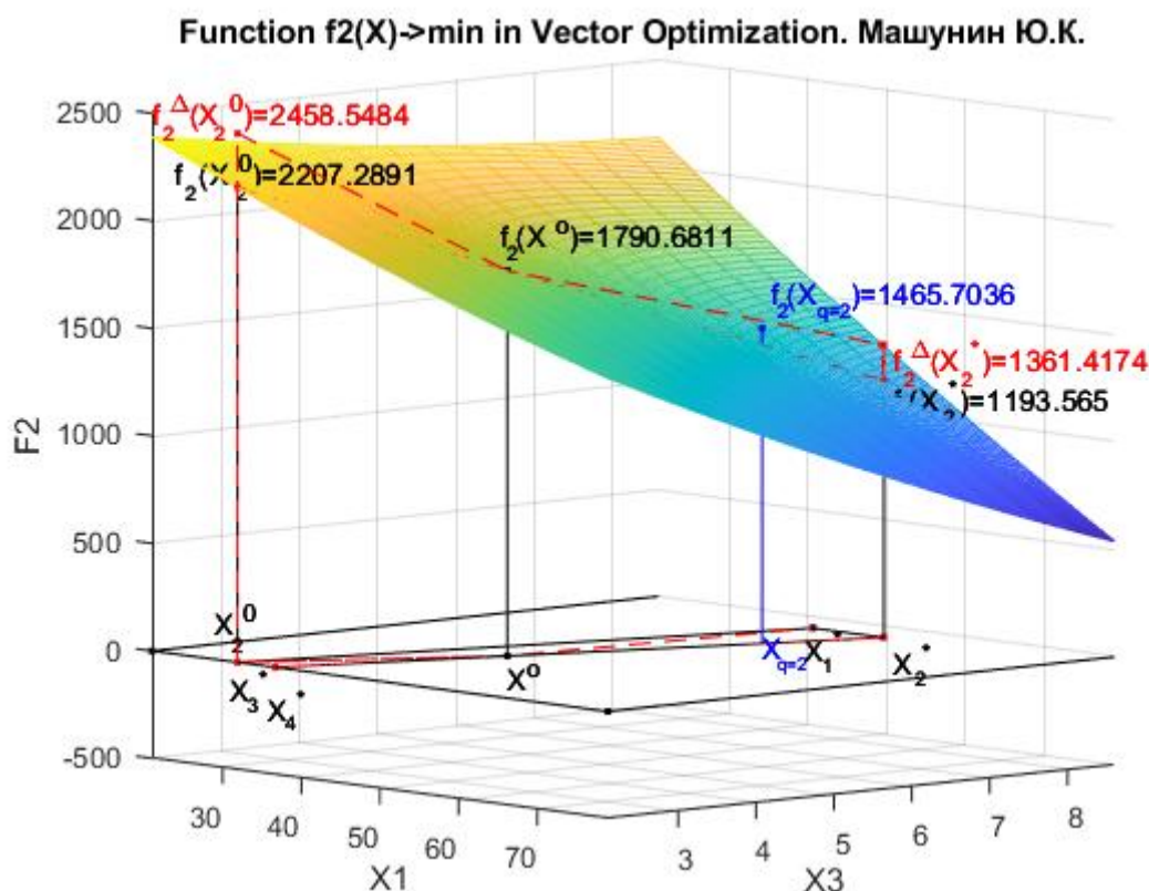
Рис. 9. Функция f_2(X) с приоритетом второго критерия в двухмерной системе координат x_1 x_3 и геометрическая интерпретация функции f_2(X) в системе координат x_1 x_2 x_3 x_4
