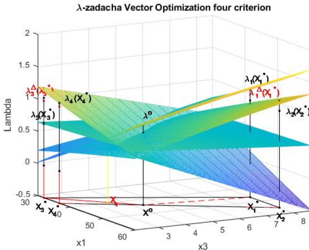
Рис. 6.2. Решение \lambda -задачи в трехмерной системе координат x_1 \ x_3 \ (= \ y_1 \ y_3) , \lambda
