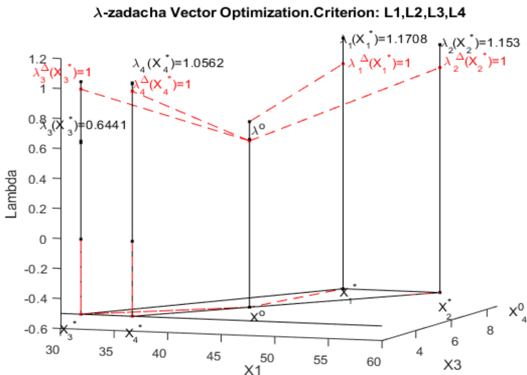
Рис. 4. \lambda -задача в системе координат x_1, x_3 (= y_1, y_3) и \lambda . Результаты решения \lambda_1(Y_1^*) = \lambda_2(Y_2^*) = \lambda_3(Y_3^*) = \lambda_4(Y_4^*) = 1; L(Y_2^*) = \{\lambda_1(Y_2^*), \lambda_2(Y_2^*), \lambda_3(Y_2^*), \lambda_4(Y_2^*)\}
