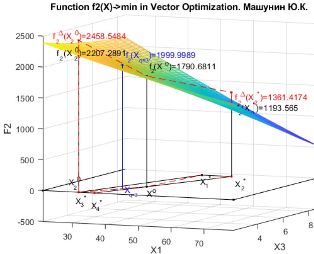
Рис. 7.k3. Функция f_2(X) с приоритетом третьего критерия в двухмерной системе координат x_1 x_3 и геометрическая интерпретация функции f_2(X) в системе координат x_1 x_2 x_3 x_4
