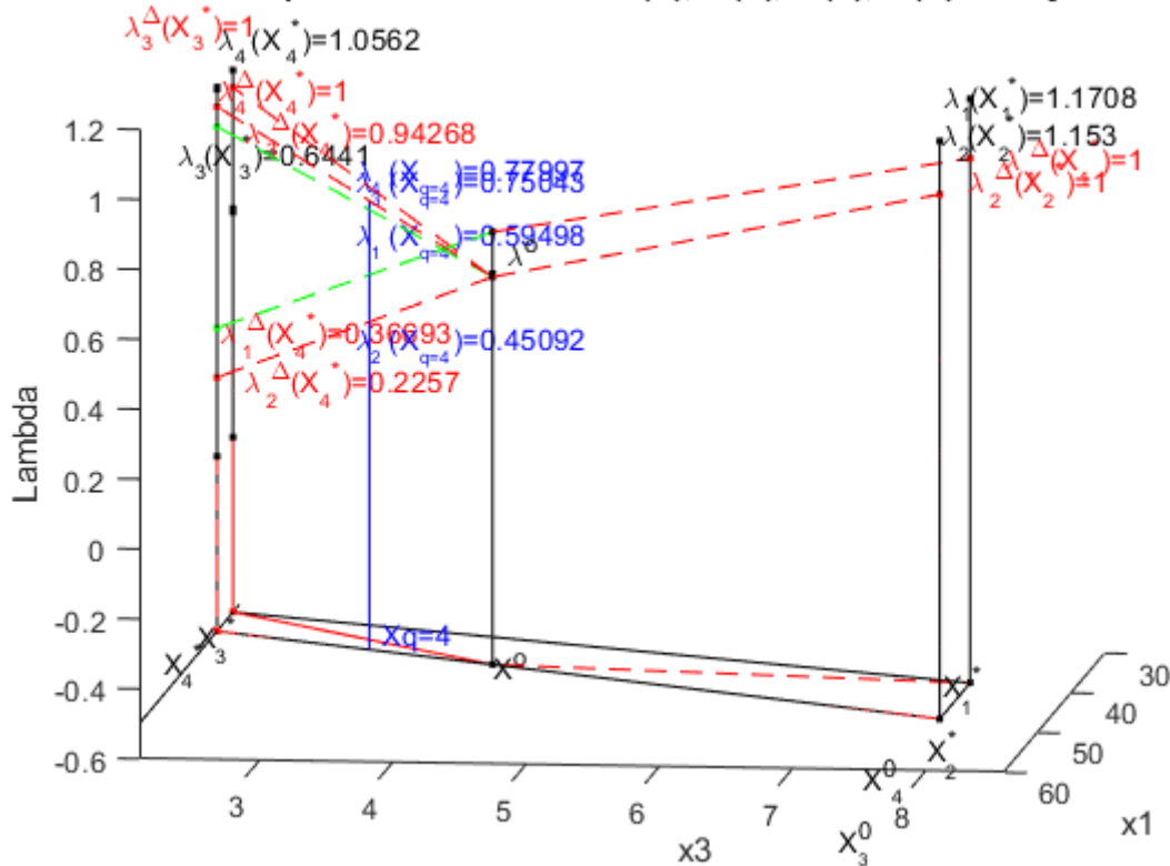
Рис. 5k3. \lambda -задача в системе координат x_1 x_3 (= y_1 y_3) и \lambda . Результаты решения:
