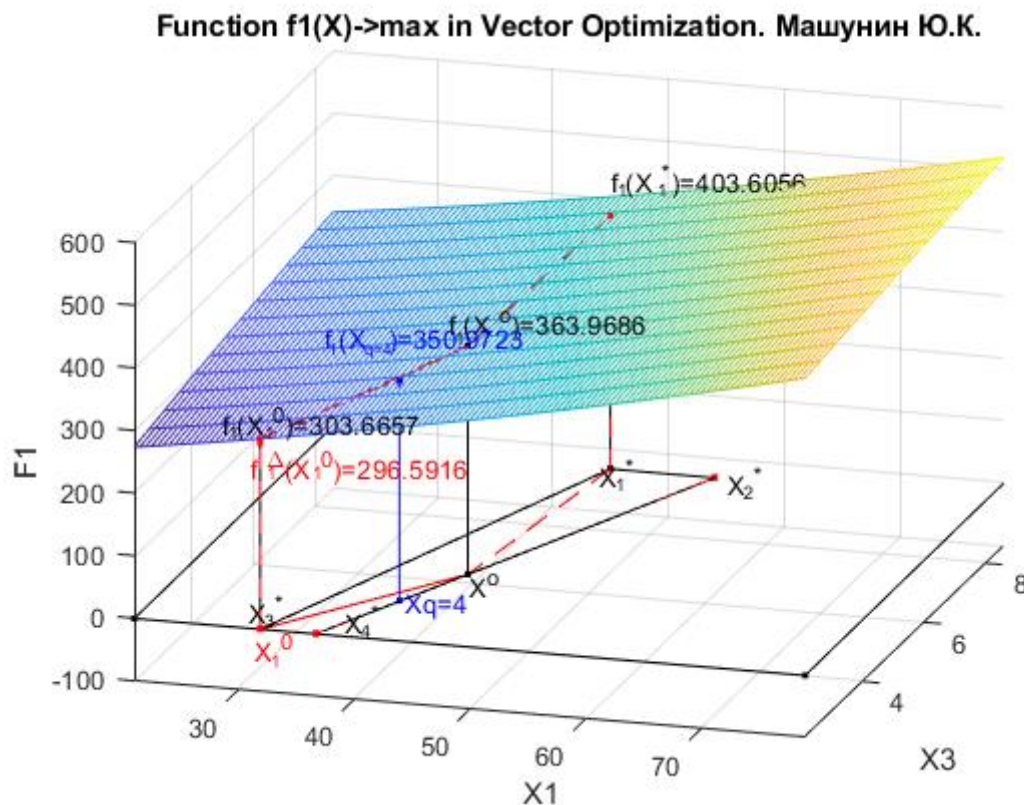
Рис. 6k4. Функция f_1(X) с приоритетом четвертого критерия в двухмерной системе координат x_1, x_3 и геометрическая интерпретация функции f_1(X) в системе координат x_1, x_2, x_3, x_4
