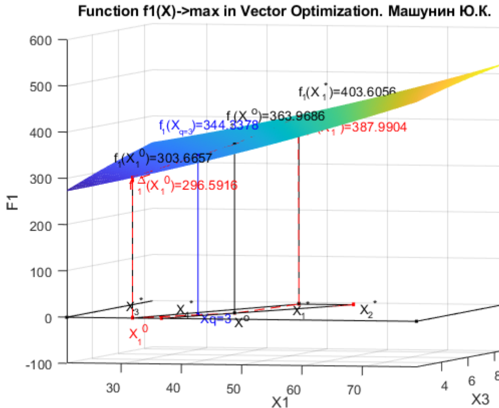
Рис. 6.к3. Функция f_1(X) с приоритетом третьего критерия в двухмерной системе координат x_1 x_3 и геометрическая интерпретация функции f_1(X) в системе координат x_1 x_2 x_3 x_4
