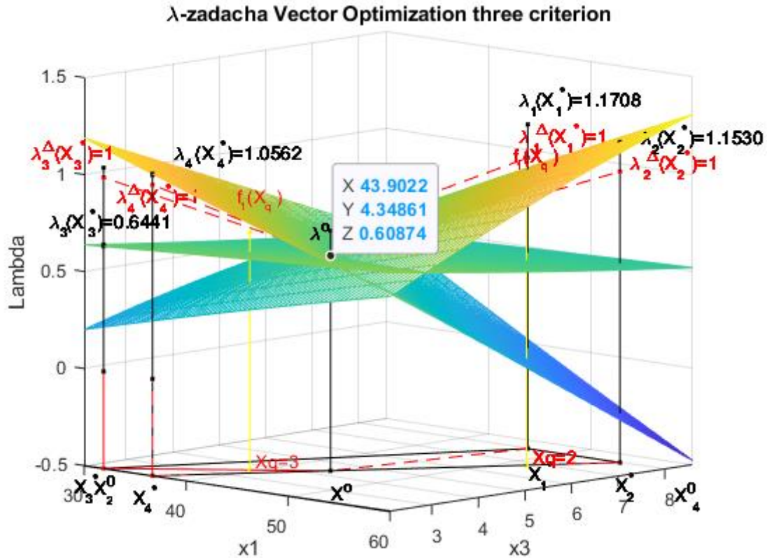
Рис. 3. Решение \lambda -задачи в трехмерной системе координат x_1, x_3 (= y_1, y_3) и \lambda
