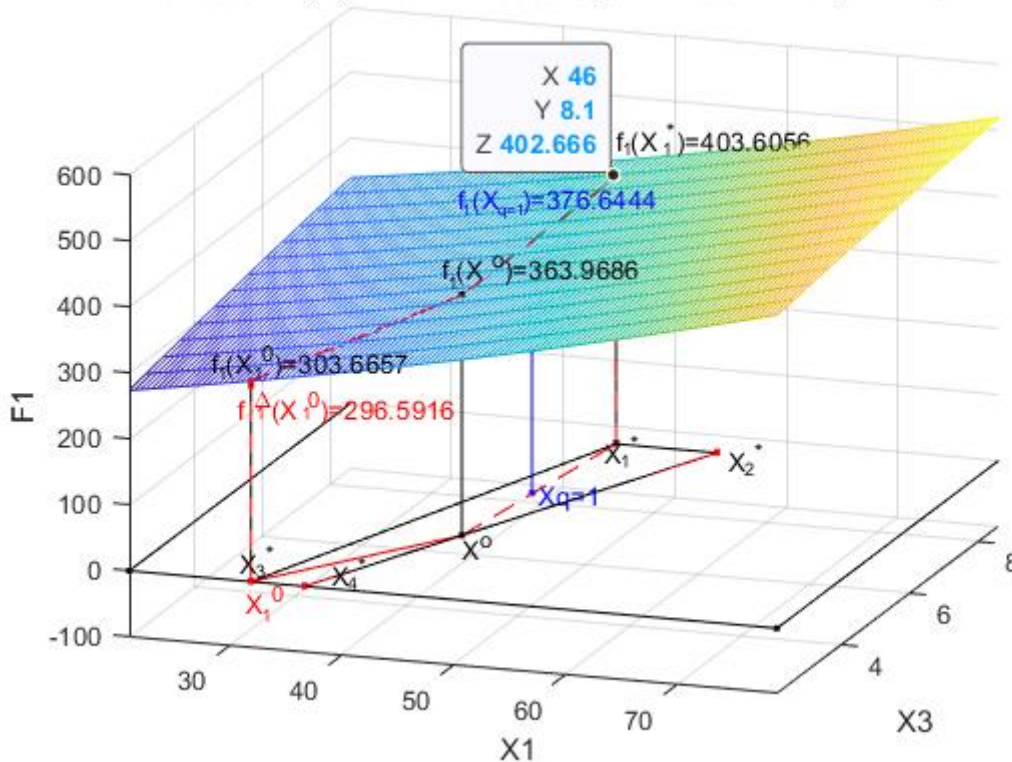
Рис. 6k1. Функция f_1(X) с приоритетом первого критерия в двухмерной системе координат x_1 x_3 и геометрическая интерпретация функции f_1(X) в системе координат x_1 x_2 x_3 x_4
