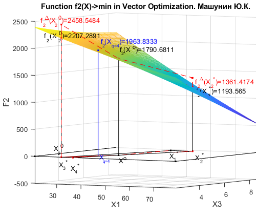
Рис. 7.k4. Функция f_2(X) с приоритетом четвертого критерия в двухмерной системе координат x_1, x_3 и геометрическая интерпретация функции f_2(X) в системе координат x_1, x_2, x_3, x_4
