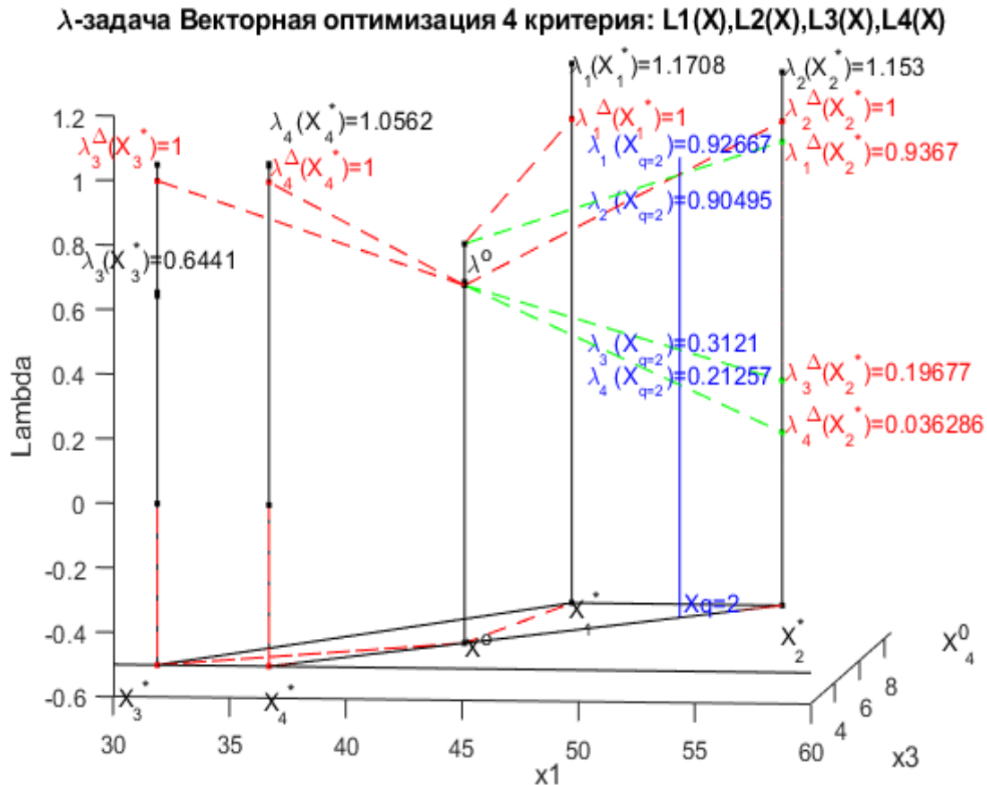
Рис. 5к2. \lambda -задача в системе координат x_1, x_3 ( = y_1, y_3 ) и \lambda . Результаты решения:
