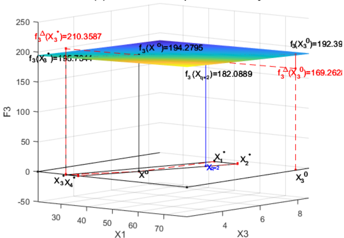
Рис. 8.k2. Функция f_3(X) с приоритетом второго критерия в двухмерной системе координат x_1, x_3 и геометрическая интерпретация функции f_3(X) в системе координат x_1, x_2, x_3, x_4
