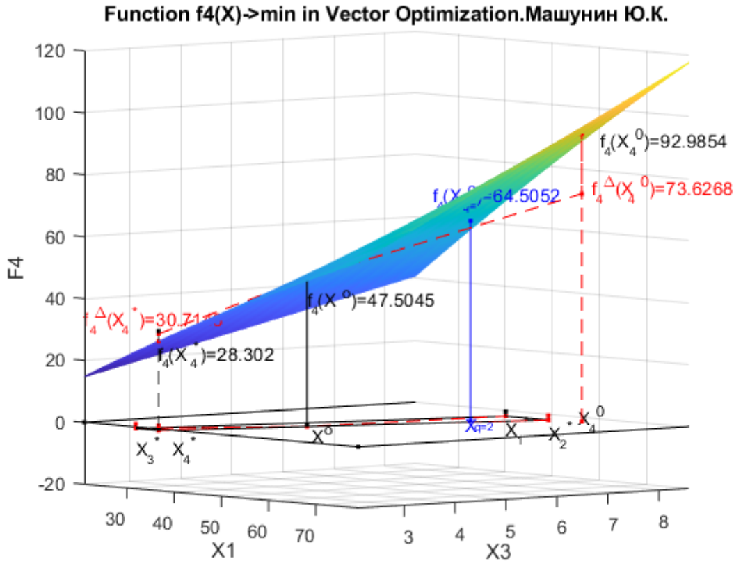
Рис. 9.k2. Функция f_4(X) с приоритетом второго критерия в двухмерной системе координат x_1, x_3 и геометрическая интерпретация функции f_4(X) в системе координат x_1, x_2, x_3, x_4
