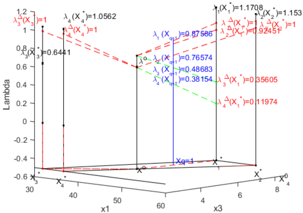
Рис. 5к1. \lambda -задача в системе координат x_1 x_3 (= y_1 y_3) и \lambda . Результаты решения:
