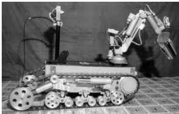
Рис. 2. Мобильный робототехнический комплекс МРК-25 (МГТУ им. Н.Э. Баумана) имеет конвертируемую ходовую часть. Складывание гусеничного обвода роботу дает возможность маневрировать в стесненных условиях (например, разворачиваться на лестничных площадках) и обеспечивает перевозку робота в джипе или микроавтобусе
